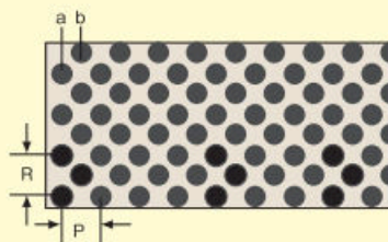
毛材配列の表現
